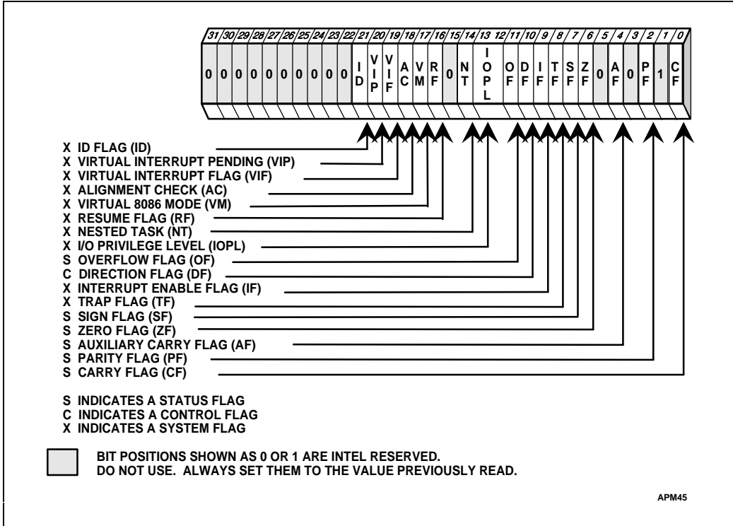
Figure 3-9. EFLAGS Register
